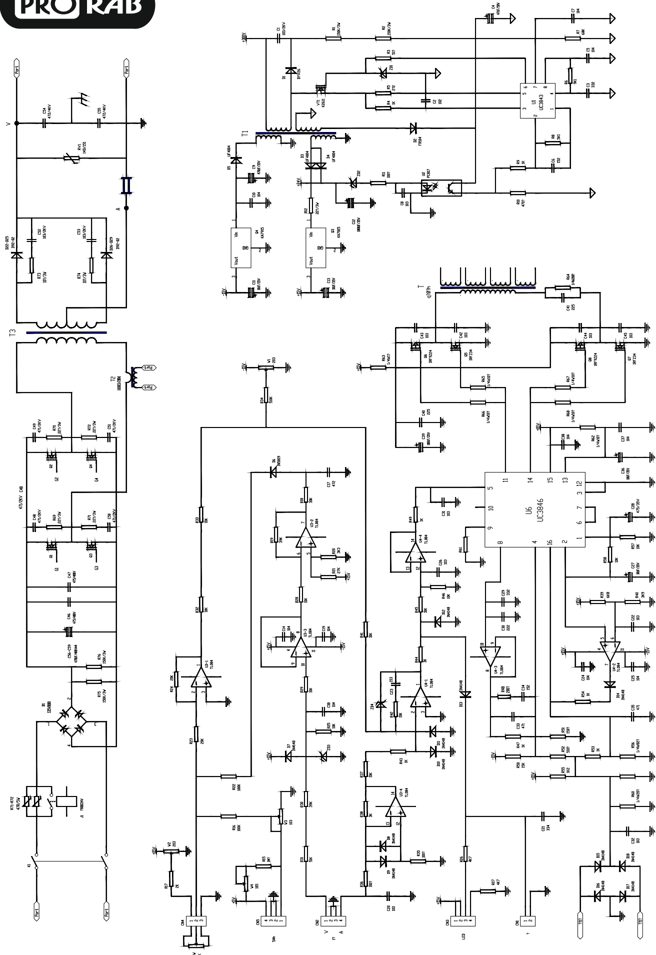
Инверторный сварочный аппарат FORWARD 200 IGBT. Электросхема.
