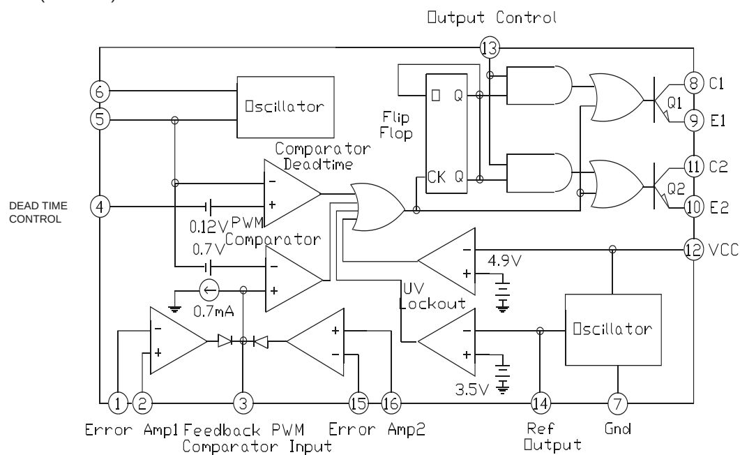
U701 (TL494CN) P.W.M IC
