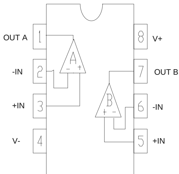
U101 (KIA4559P) - DUAL OP AMP U111,702 (KIA393P)
