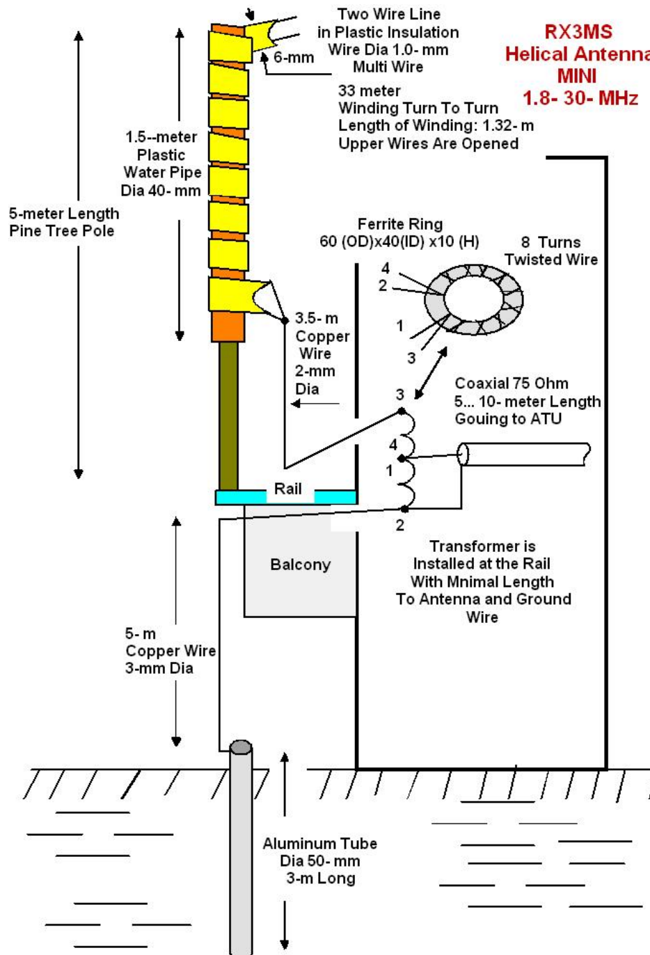
Figure 3 MINI RX3MS Helical Antenna
