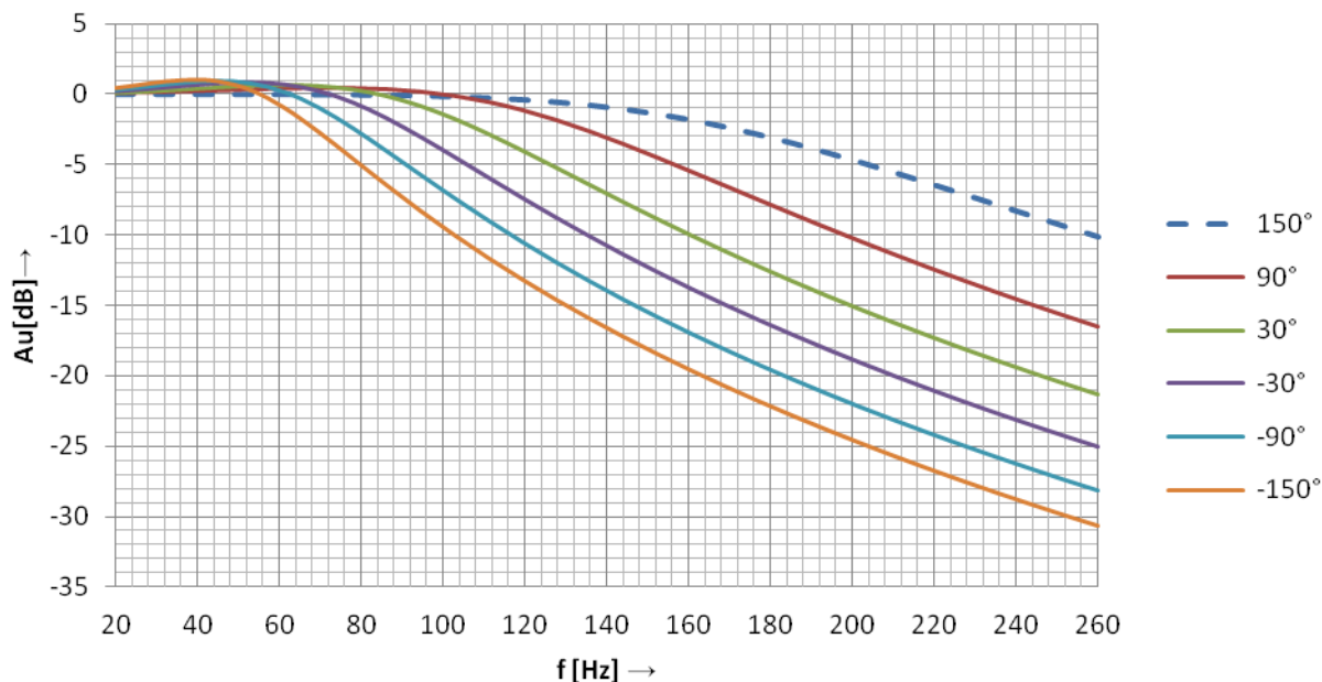
Obrázek 2.6: Simulace nastavitelné dolní propusti
