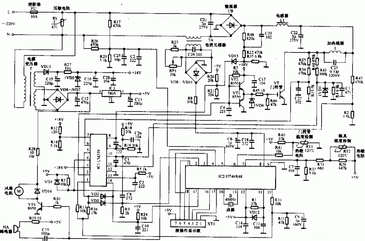
图 1-15 富士电 IH-P190B 电磁炉控制板电路图
