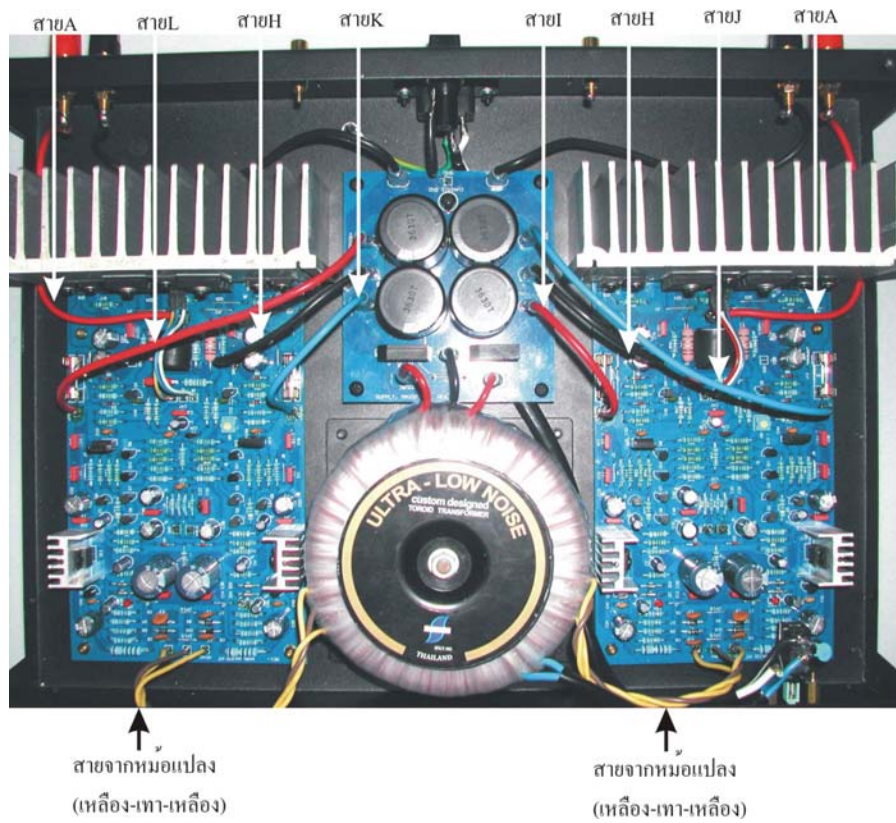
รูปที่ 35 การต่อสายไฟและเอาต์พุต
