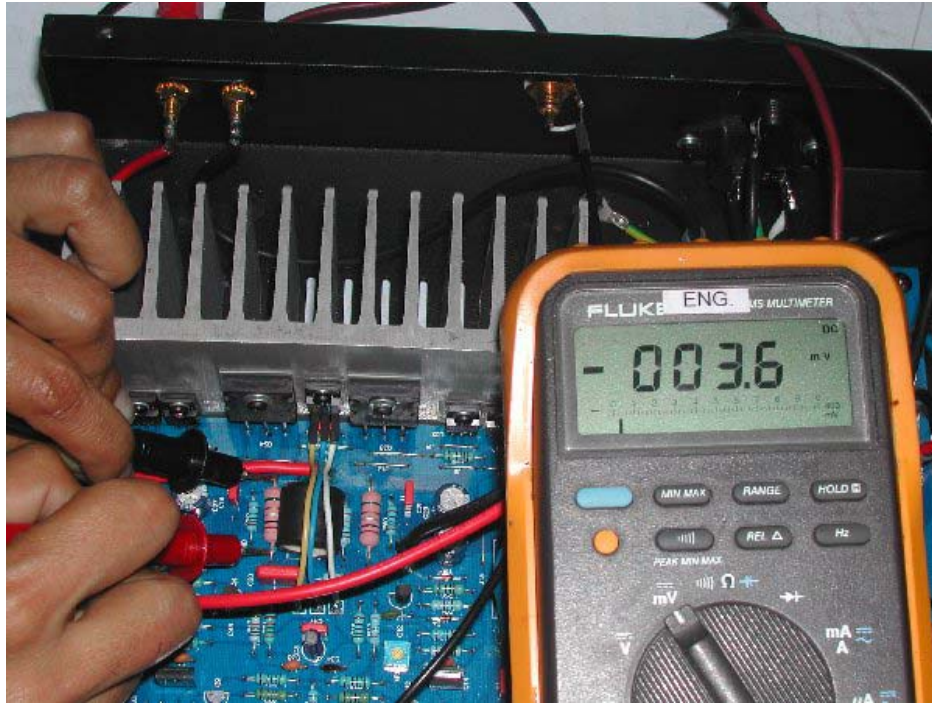
รูปที่ 40 แสดงการปรับกระแสสงบ(กระแส Idle)
