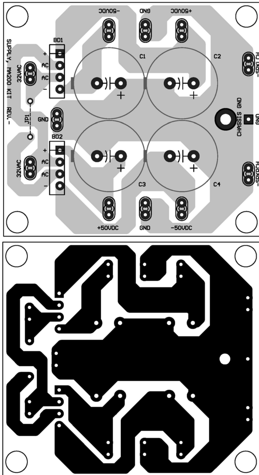
รูปที่ 12. layoutของแผง และด้านใส่อุปกรณ์ของแผ่น Power Supply Board
