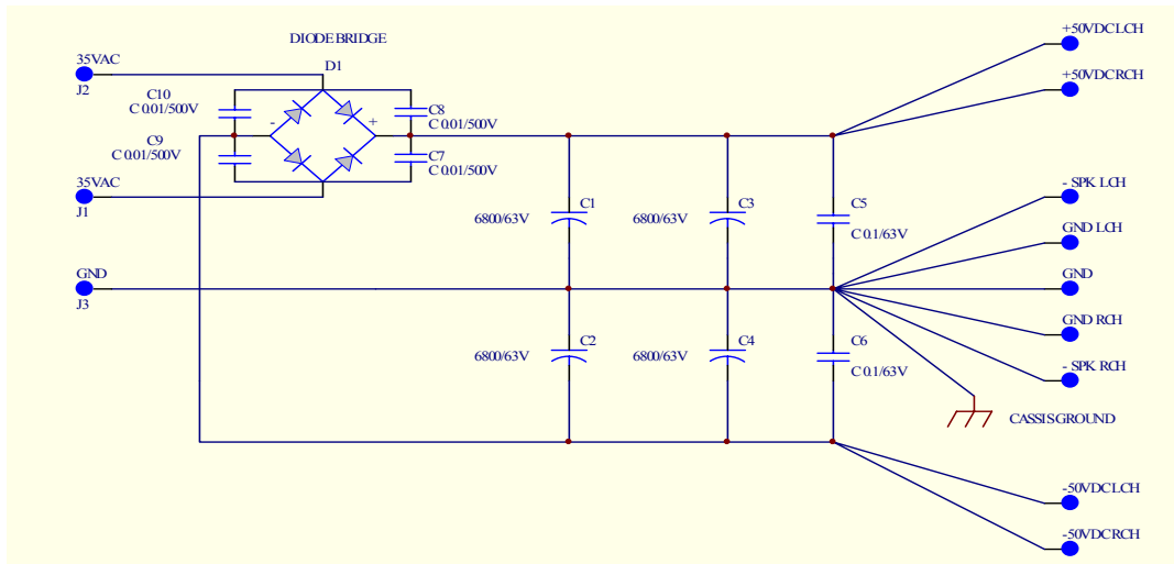
ข. วงจรภาคจ่ายไฟแบบ unregulate
