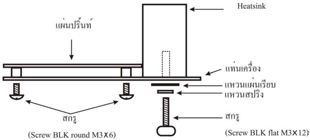
รูปที่ 34 การยึด Heatsink เข้ากับแท่นเครื่อง
