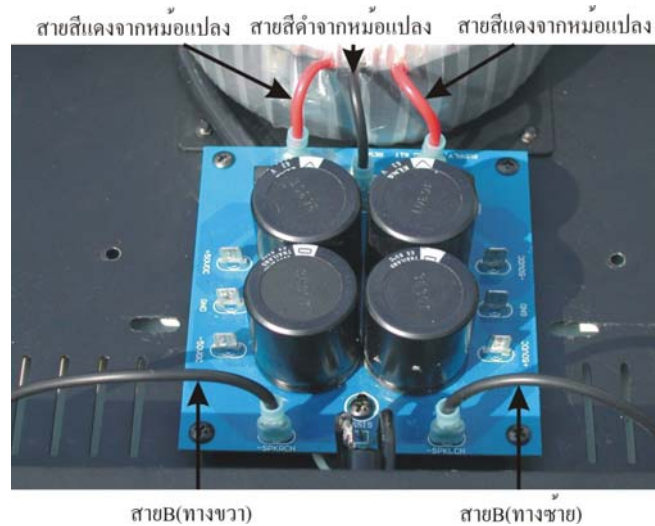
รูปที่ 32 การต่อสายไฟเข้าสู่ชุดจ่ายไฟ
