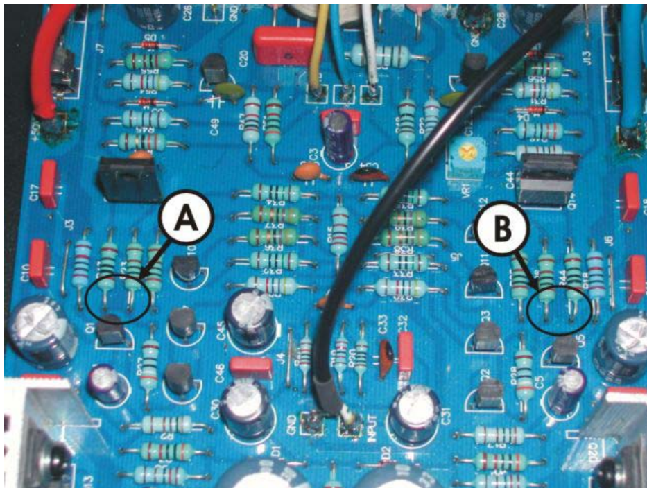
รูปที่ 39 จุดวัดไฟ A และ B
