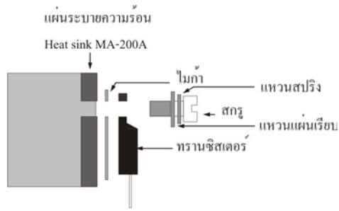
รูปที่ 17 การยึดตัวทรานซิสเตอร์ติดกับฮีทซิงค์
