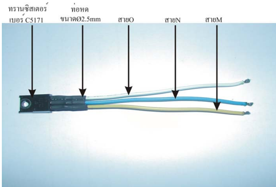
รูปที่ 19 การต่อขาของตัวทรานซิสเตอร์Q15
