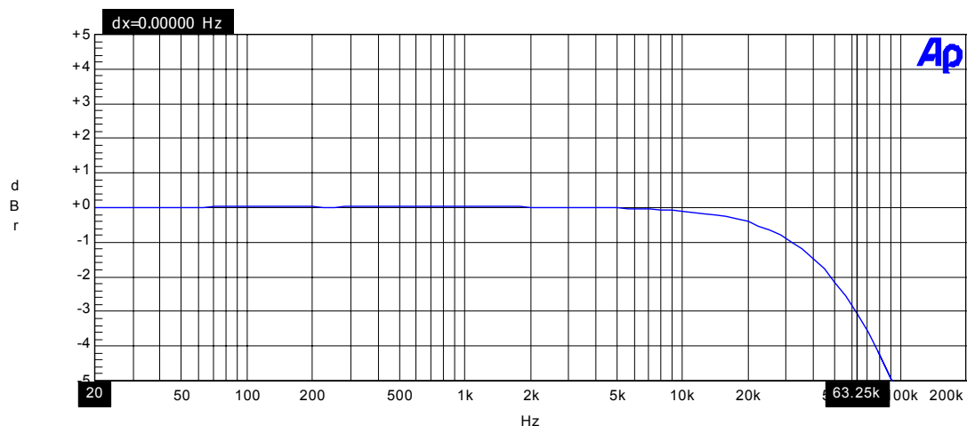
รูปที่ 3 เป็นกราฟแสดงผลการตอบสนองความถี่ที่ -3 dB
