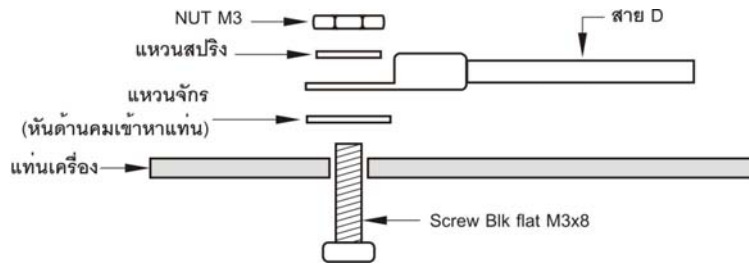
รูปที่ 25 แสดงการยึดสาย D ลงแทน
