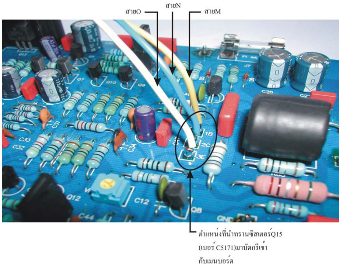
รูปที่ 20 ตำแหน่งที่ต่อขาของทรานซิสเตอร์
