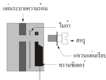
รูปที่ 13 การยึดทรานซิสเตอร์ Q13 และ Q20 เข้ากับแผ่นระบายความร้อน
