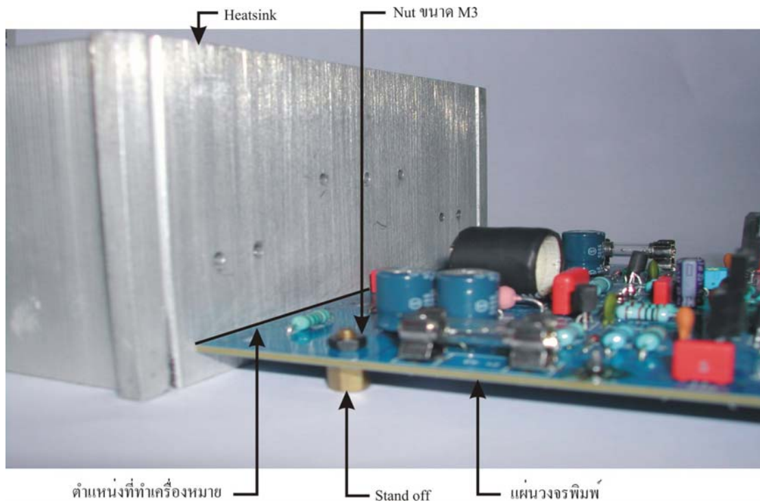
รูปที่ 14 การวางแผ่นวงจรพิมพ์บน Stand off
