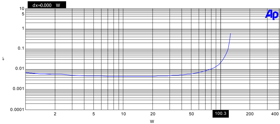
รูปที่ 4 เป็นการวัดค่า THD โดยเริ่มทำการ Sweep ตั้งแต่ 1 Wrms ถึงกำลังขับสูงสุด ความถี่ 1KHz ที่โหลด 8Ω จากกราฟแสดงให้เห็นว่า Power Amplifier สามารถขับโหลด 8Ω ได้ 100Wrms ก่อนที่จะเกิดการ Clip ซึ่งการ Clip นี้จะทำให้เกิด THD เกินกว่าที่จะยอมรับได้ (สังเกตว่าที่กำลังงานสูง THD จะเพิ่มขึ้นเพราะวงจร Harmonic Reduction เริ่มทำงาน)
