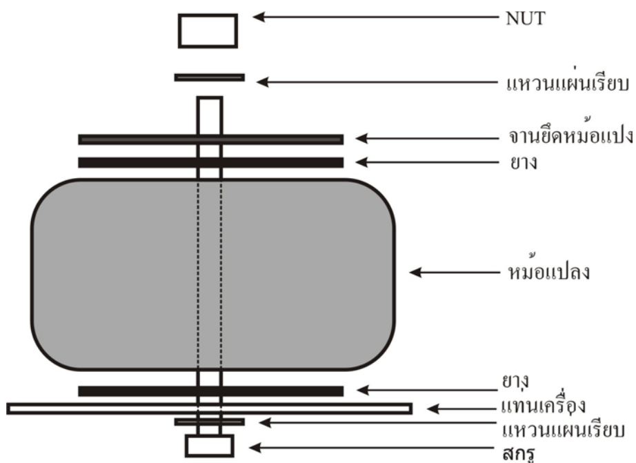
รูปที่ 29 การยึดหม้อแปลง
