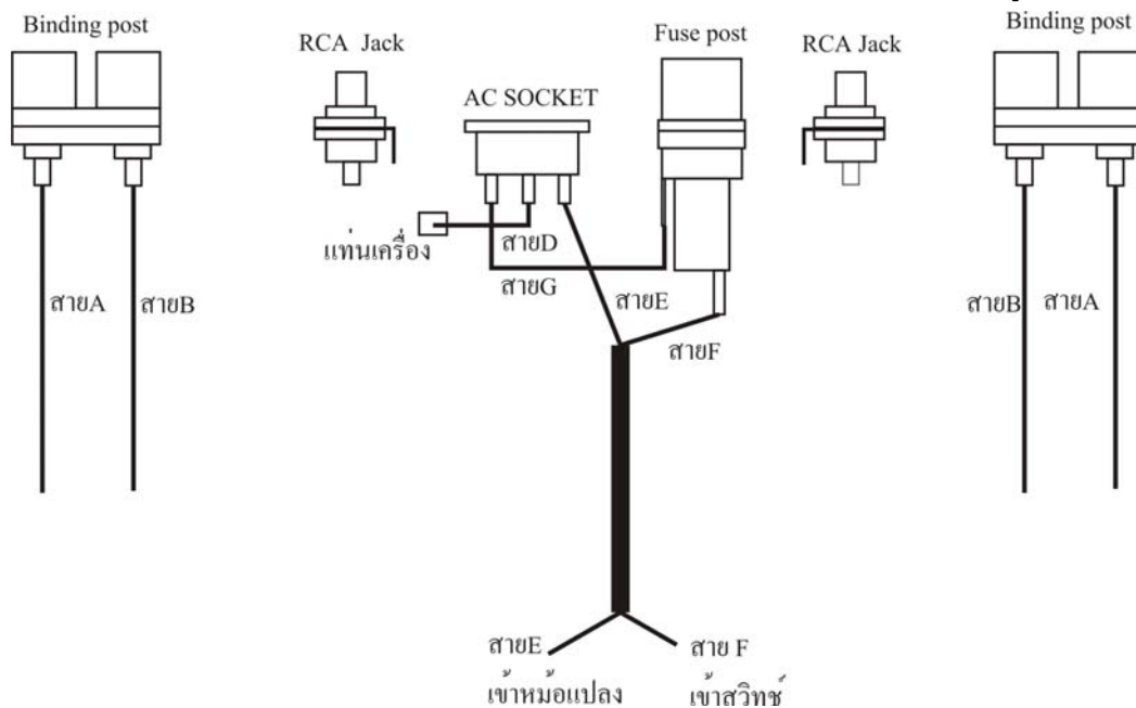
รูปที่ 24 การต่อสายที่อุปกรณ์หลังเครื่อง
