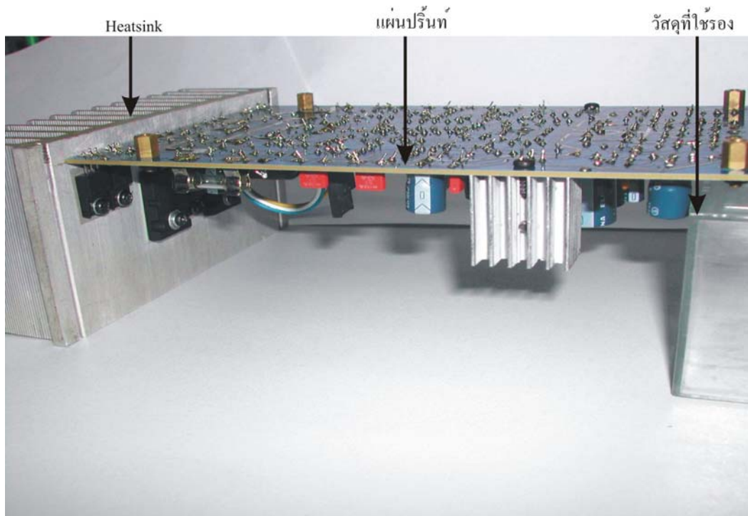
รูปที่ 18 การวางแผ่นปริ้นท์ก่อนการบัดกรีขาตัวทรานซิสเตอร์
