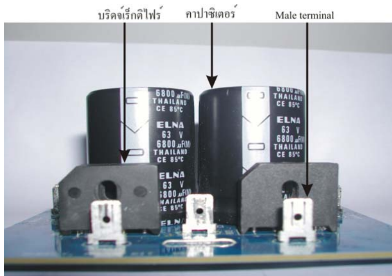
รูปที่ 22 แสดงการลงอุปกรณ์บนแผ่นปริ้นท์ของ Power Supply
