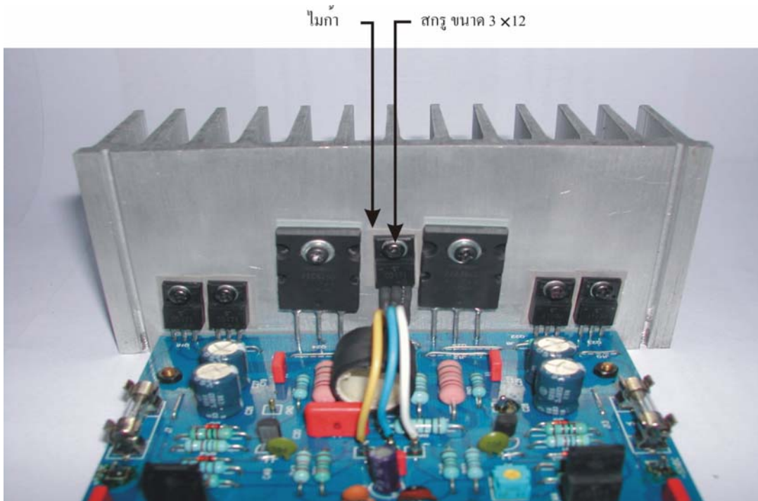
รูปที่ 21 การยึดตัวทรานซิสเตอร์ที่มีการต่อขา
