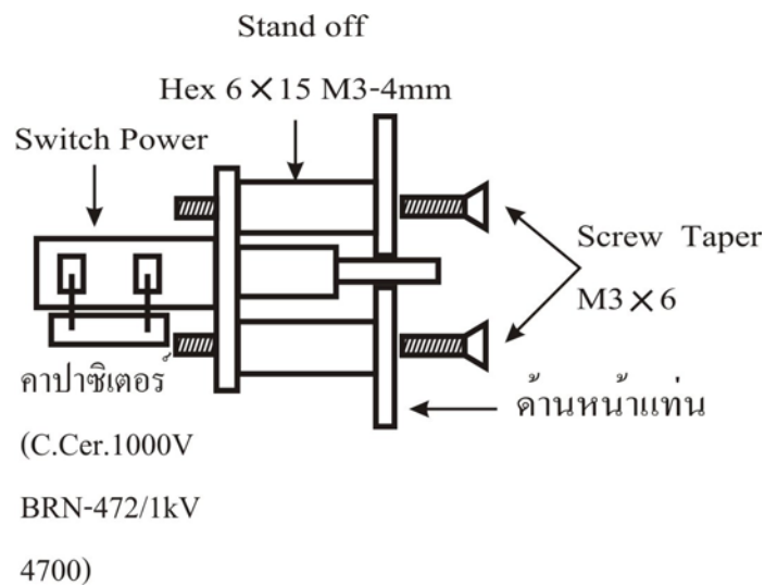
รูปที่ 26 การติดตั้งสวิตช์เพาเวอร์ที่ด้านหน้าแทน
