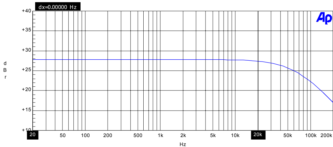
รูปที่ 2 เป็นกราฟแสดงผลการตอบสนองของความถี่ตั้งแต่ช่วง 20Hz-20kHz
