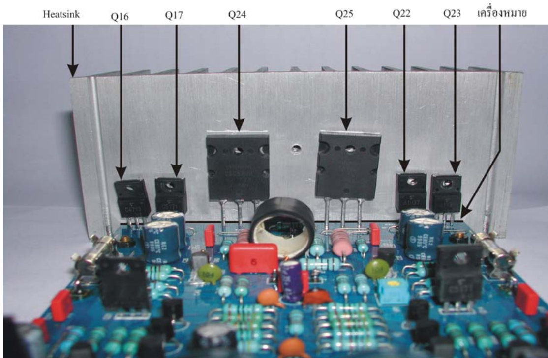
รูปที่ 15 การวางตัวทรานซิสเตอร์ลงบนแผ่นวงจรพิมพ์
