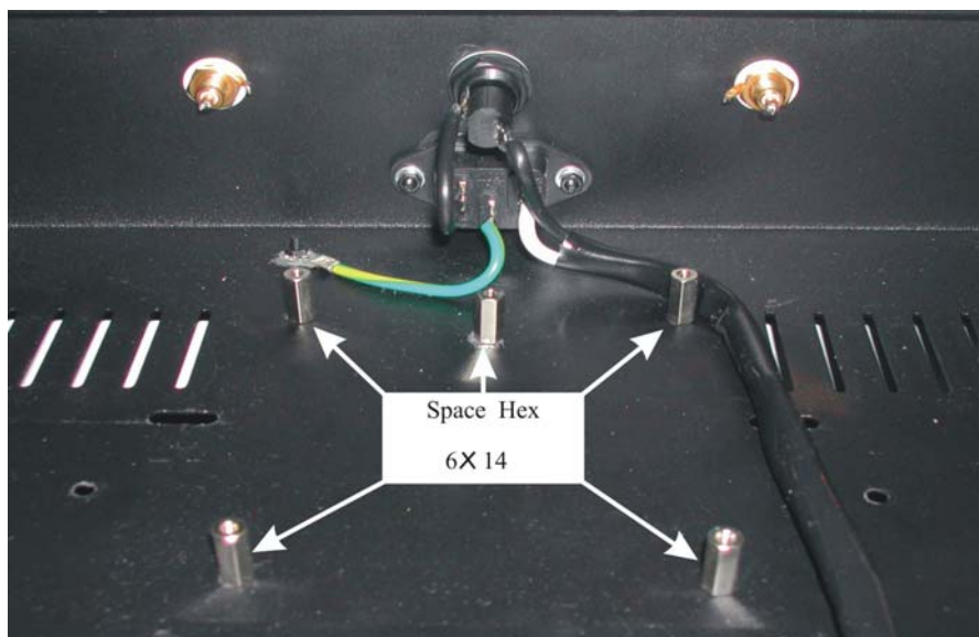
รูปที่ 27 การติดตั้ง Spacer Hex 6x14,M3
