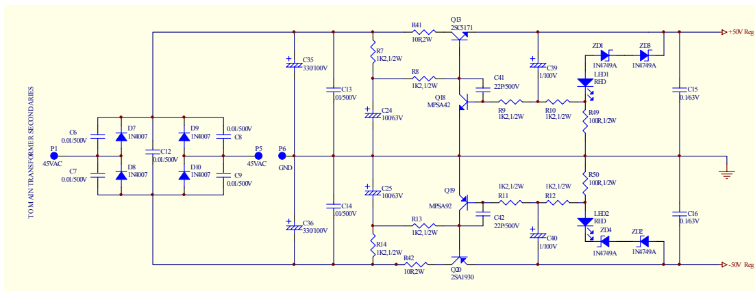
ก. วงจรภาคจ่ายไฟ แบบ Regulate
