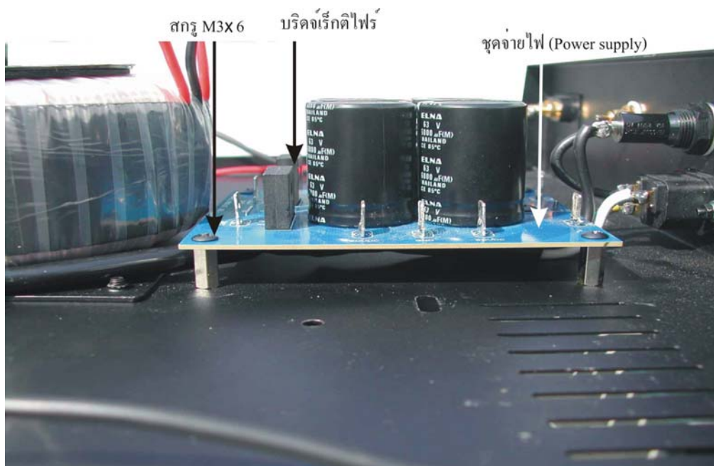
รูปที่ 31 การติดตั้งชุดจ่ายไฟ
