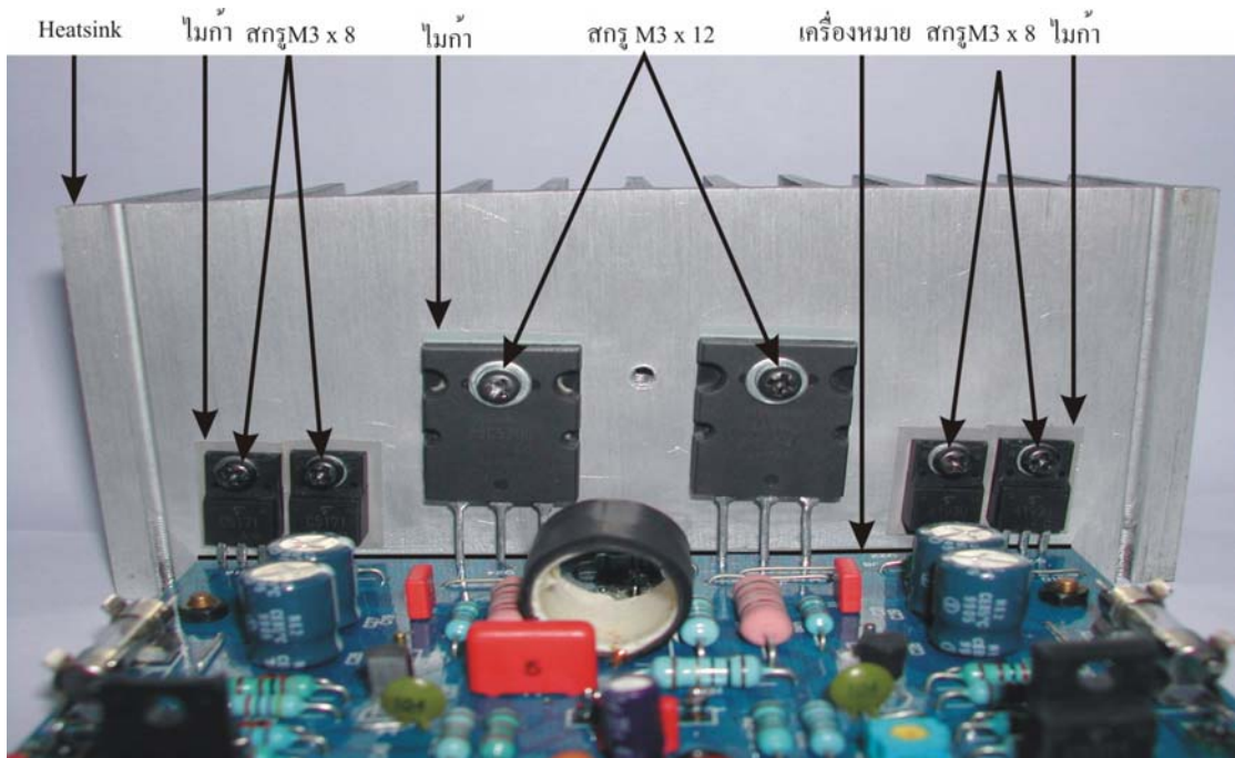
รูปที่ 16 การยึดตัวทรานซิสเตอร์กับHeatsink
