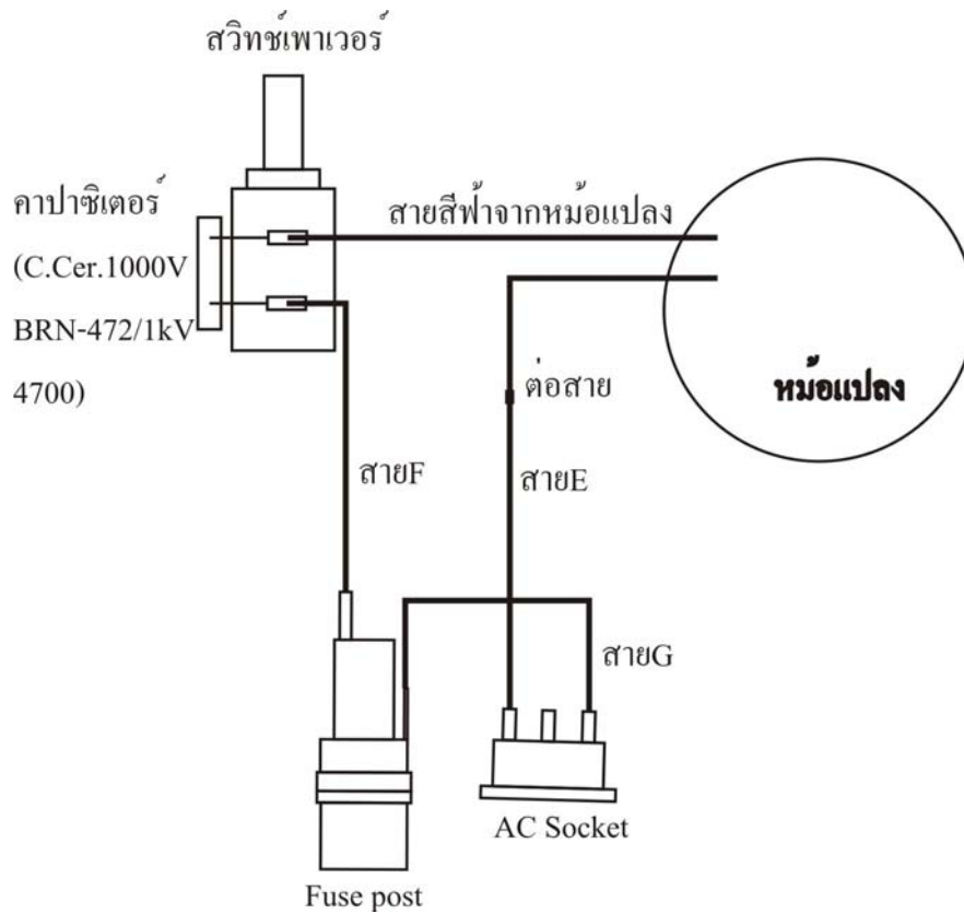
รูปที่ 30 การต่อสวิตช์เพาเวอร์
